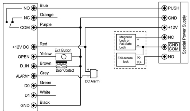
schema alimentazione elettrica del controllo accessi
