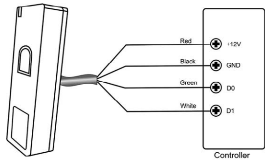
schema di collegamento come lettore collegato a controller esterno
