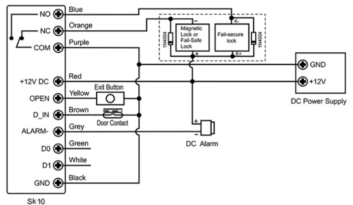
schema alimentazione elettrica del controllo accessi
